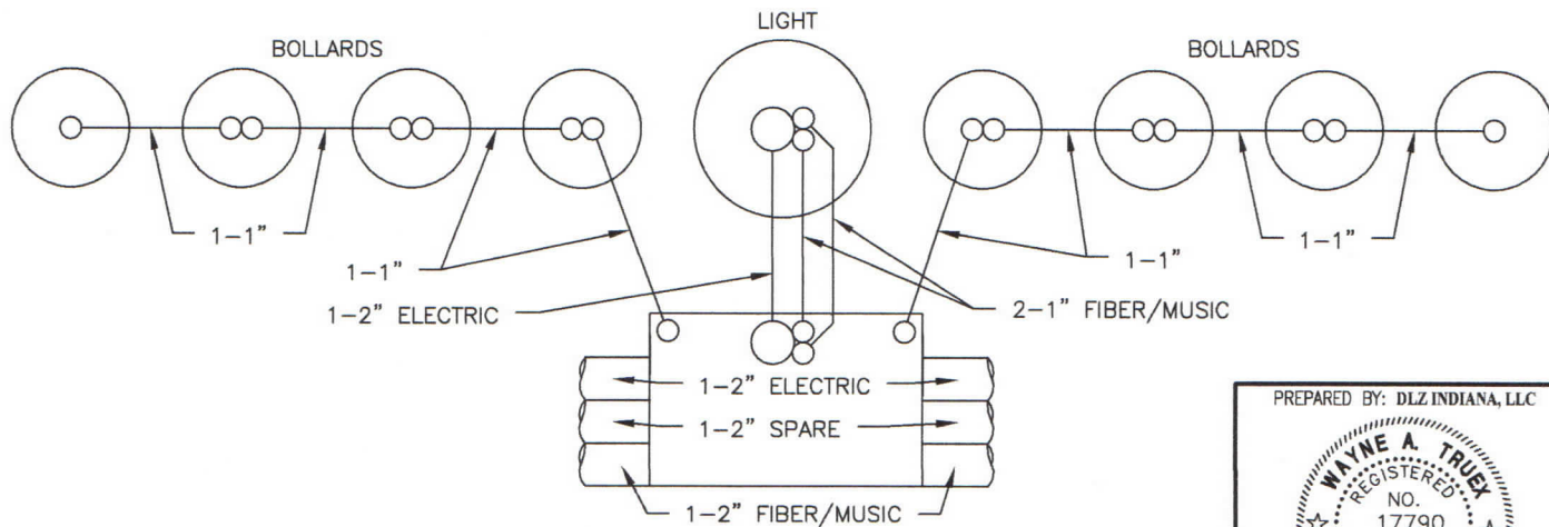
LIGHTED BOLLARD HANDHOLE N.T.S.
