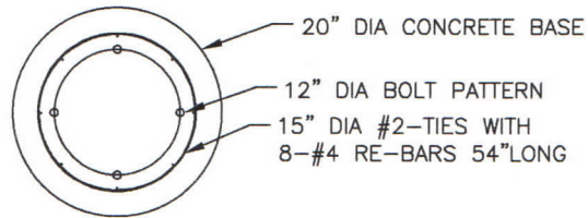
PLAN VIEW N.T.S.
