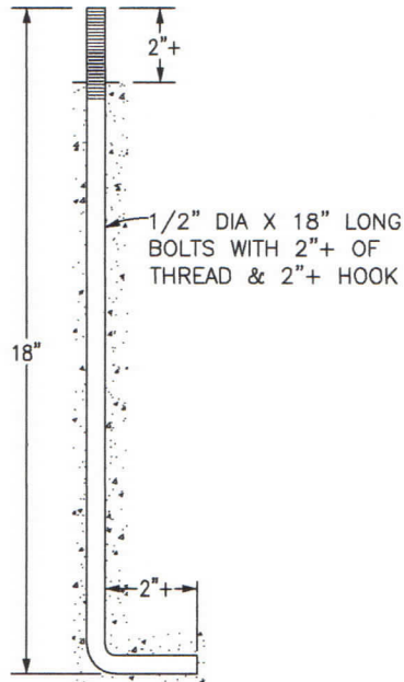
ANCHOR BOLT N.T.S.
