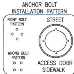
PLAN VIEW N.T.S.
