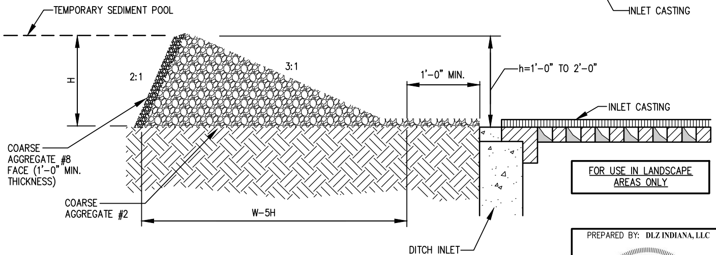
SECTION A-A
